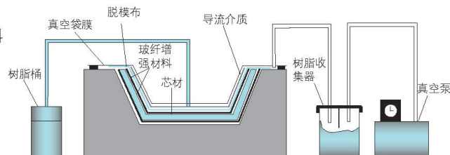
真空导入成型示意图
